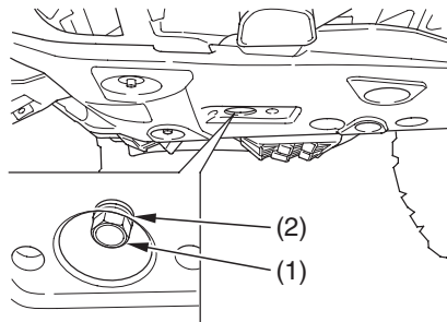
(1) moottoriöljyn tyhjennystulppa (2) tiiviste
