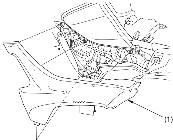
(1) vasen sivusuoja
