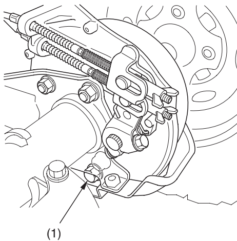
(1) takajarrun tyhjennyspultti
